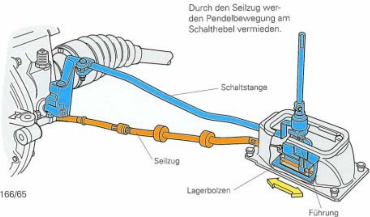
Schaltung mit Seilzug
